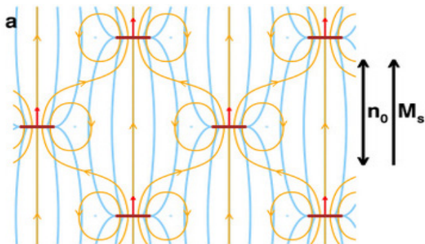
Shematski prikaz ukrivljenosti direktorja tekočega kristala (modro) in magnetnega polja (rumeno) okrog magnetnih ploščic (pogled od strani, rdeče vodoravne črte) s smerjo magnetnega momenta pravokotno na ploščice (rdeče puščice)
